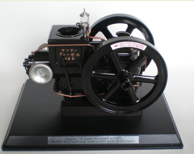
世界初の小型ディーゼルエンジン「HB型」1933年
